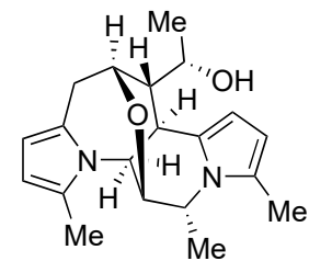
(±) Bipolarine I
